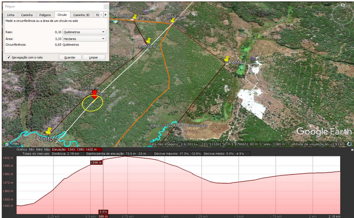
Figura 9: Mapa de elevação no sentido latitudinal norte-sul, com uma diferença de cota entre os 1343 e 1402 m de 73,5 m distribuídos em uma distância de 2,19 km, com inclinação máxima de 17,3 % e média de 5%. Há necessidade de aplicação de medidas anti erosivas em mais 3,3 ha.
