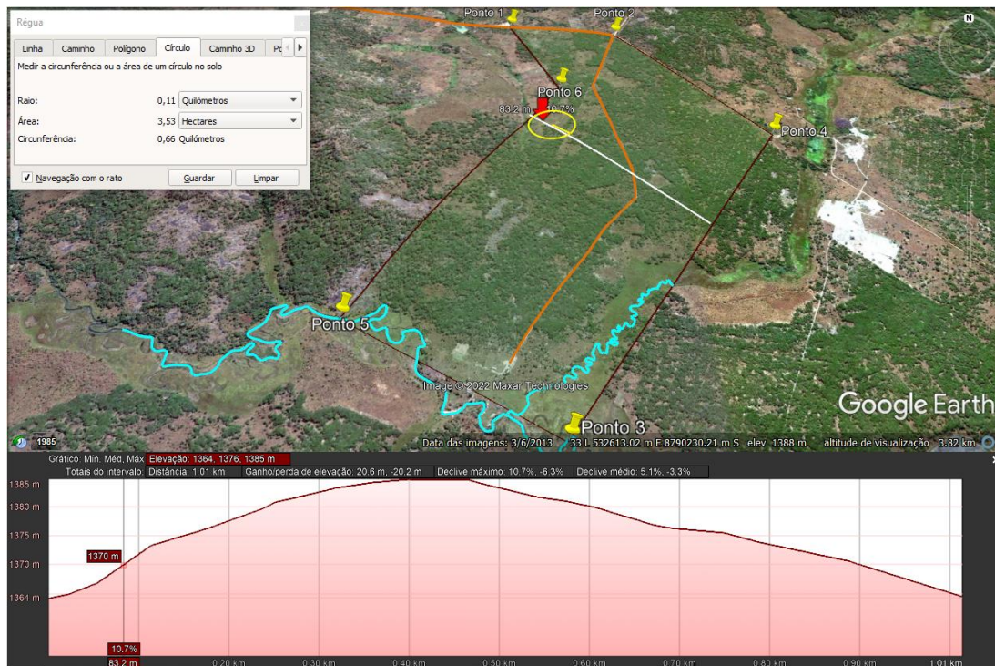
Figura 11: Mapa de elevação na parte cento-norte da propriedade, no sentido longitudinal oeste-este, com uma distância de 1,01 km, há uma diferença de cota entre os 1364 e 1385 m pelo ganho de elevação em 20,6 m e perda de -20,2 m, com declive máximo de 10,7 % e médio de 5,1%, o que solicita a aplicação de medidas anti erosivas em 3,53 ha.
