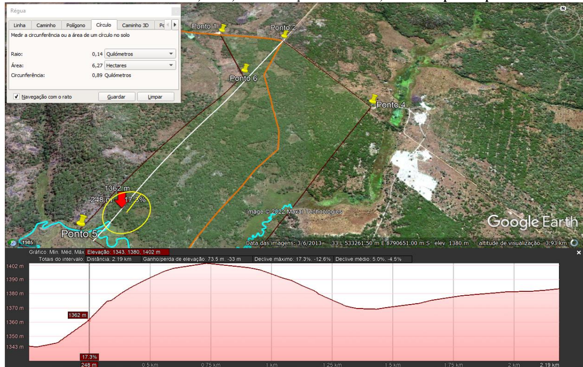
Figura 8: Mapa de elevação no sentido latitudinal norte-sul, na parte mais alta da Fazenda, há uma diferença de cota entre os 1343 e 1402 m de 73,5 m distribuídos em uma distância de 2,19 km, com inclinação máxima de 17,3 % e média de 5%. Há necessidade de aplicação de medidas anti erosivas em cerca de 6,27 ha.
