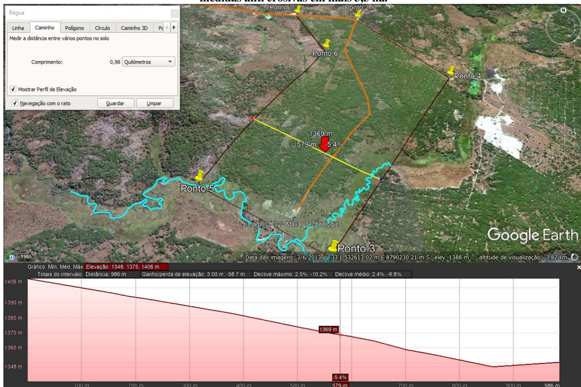
Figura 10: Mapa de elevação na parte centro-sul da propriedade, no sentido longitudinal oeste-este, com uma distância de 0,986 km, há uma diferença de cota entre os 1348 e 1406 m pelo ganho de elevação em 3 m e perda de -58,8 m, com declive máximo de 2,5 % e médio de 2,4%. Dispensa-se a aplicação de medidas anti erosivas.
