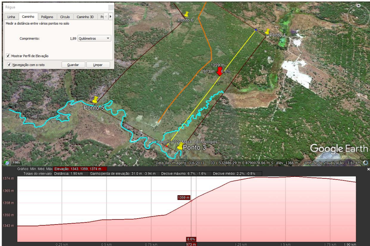
Figura 7: Mapa de elevação no sentido latitudinal norte-sul, na zona do terço, há uma diferença de cota de 31 m entre os 1343 e 1374 m distribuídos em uma distância de 1,90 km, com inclinação máxima de 6,7 % em um ponto específico e média de 2,2%.
