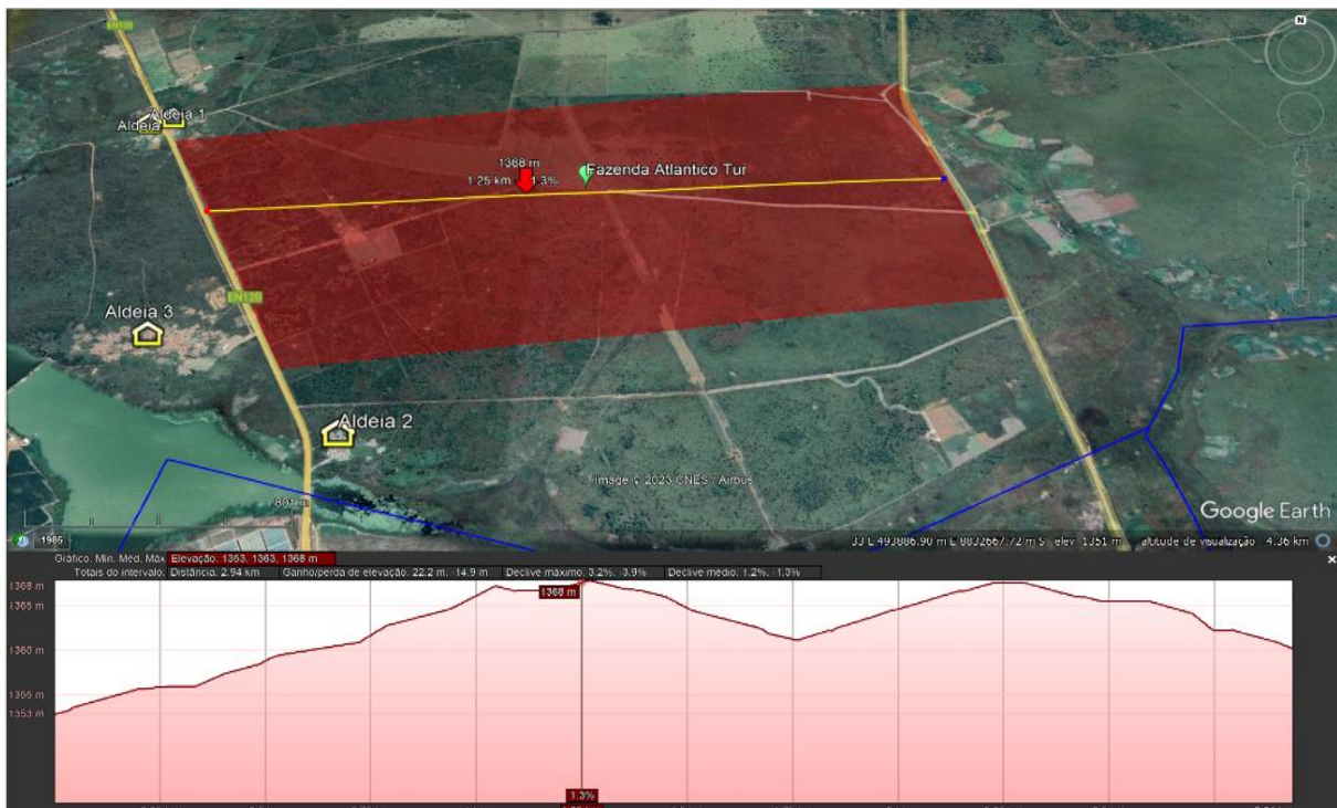
Figura 2: Sentido Este –Oeste ao centro do terreno, numa distância de 2,94 km, a elevação tem uma variação de 22,2 m (-14,9 m), com inclinação máxima de 3,2% (-3,9%) e uma inclinação média de 1,2% (-1,3%). As medidas anti erosivas devem ser implementadas de 1,5 km até 2,25 km e de 2,5 km á 2,94 km
